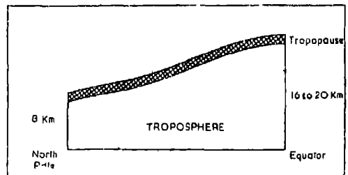
Fig. 57. Troposphere
