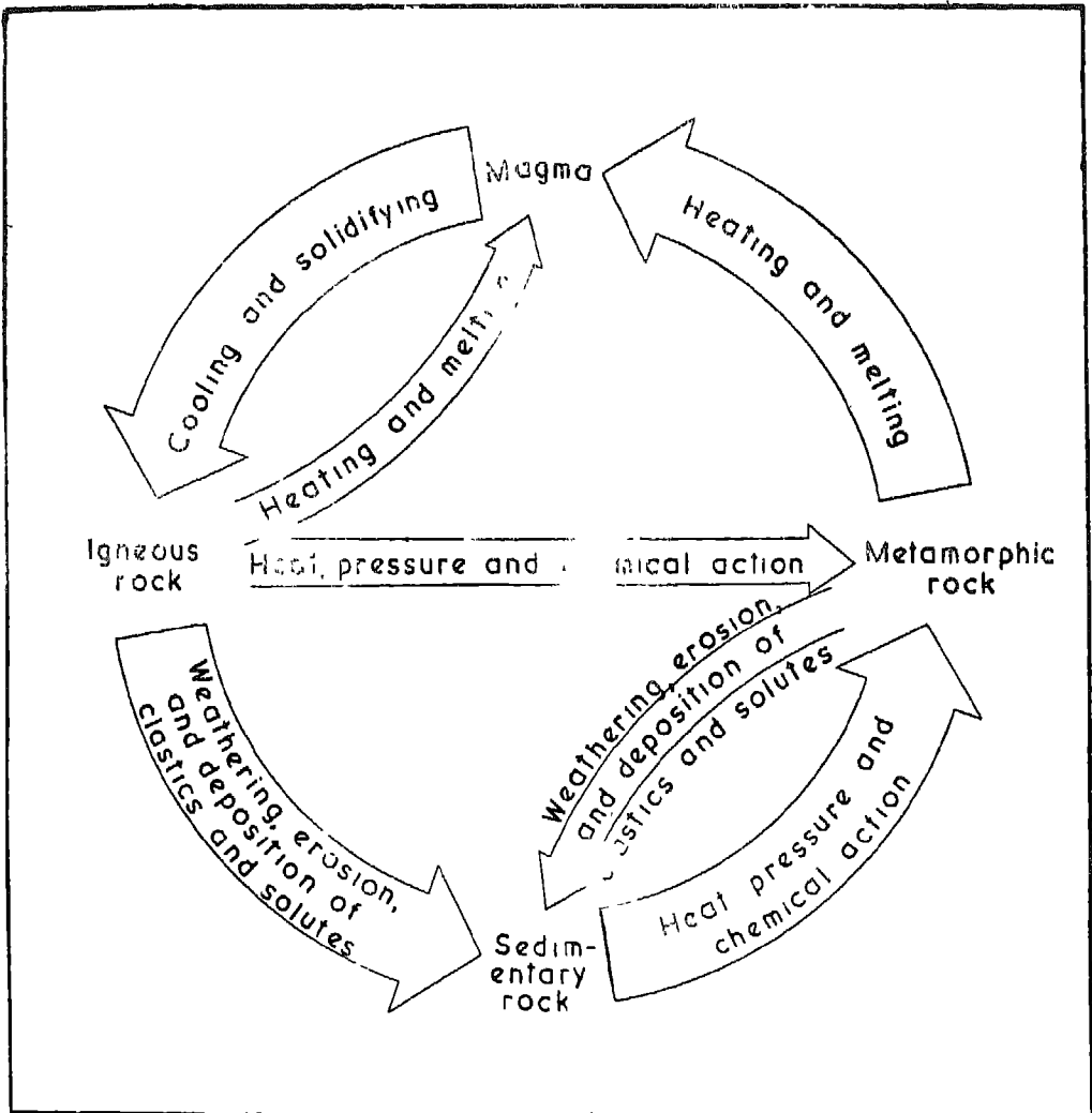
Fig. 18. Rock Cycle
