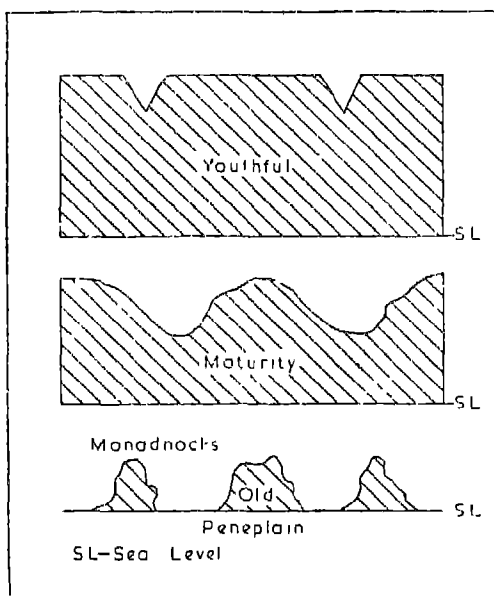
Fig. 28. Fluvial Cycle
